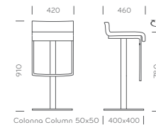
Colonna Column 50x50 | 400x400 | Meccanismo di ritorno automatico With automatic spring back device
