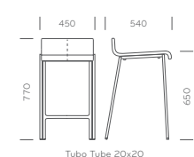
Tubo Tube 20x20
