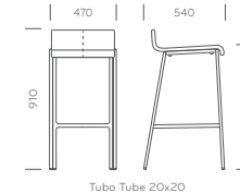
Tubo Tube 20x20
