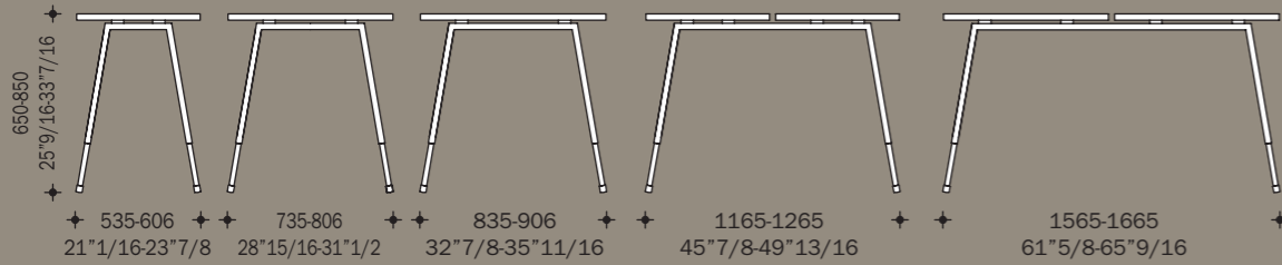
P551921 Gamba a ponte / Straight leg / Piètement droit / Pata recta
