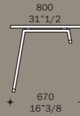
P551912 Gamba a cavalletto regolabile / Adjustable A-shape leg / Piètement trèteau réglable en ht. / Pata de caballete regulable en altura
